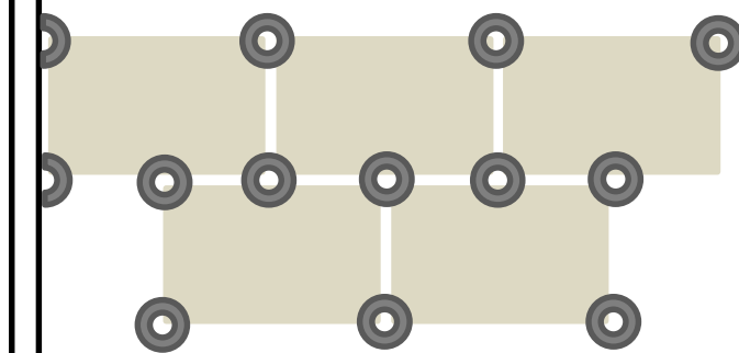
Plattenformate mit versetzter Fuge: 30x60, 40x50, 40x60, 40x70, 50x70, 60x40
