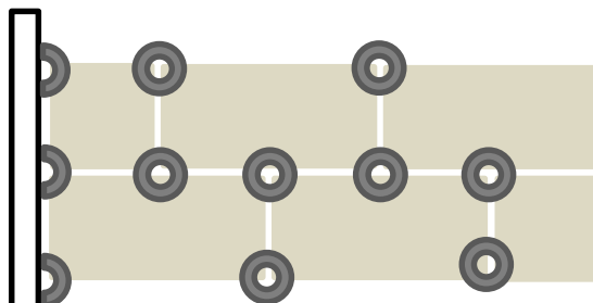
Plattenformate mit versetzter Fuge: 30x60, 40x50, 40x60, 40x70, 50x70, 60x40
