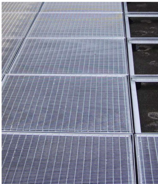
Abb. 22: PLV50/75 mit ZSt65/100 unter Gitterplatten, 135-170 mm.
