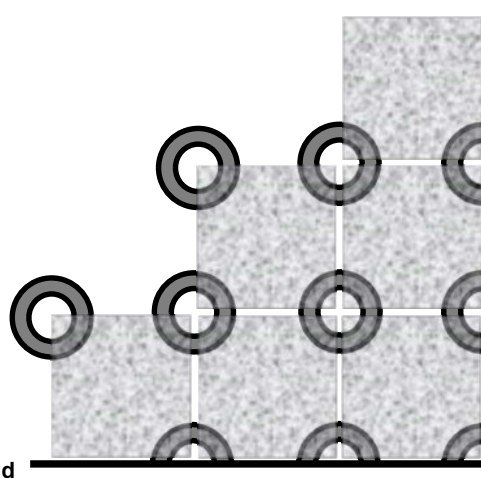
Abb. 5: Randverlegung: Schematische Darstellung einer Randverlegung mit starren Stelzlager.
