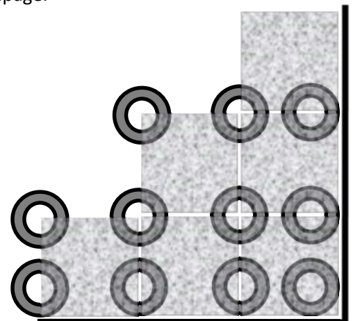
Abb. 12: Randverlegung: Schematische Darstellung einer Randverlegung mit höhenverstellbaren Stelzlagern.
