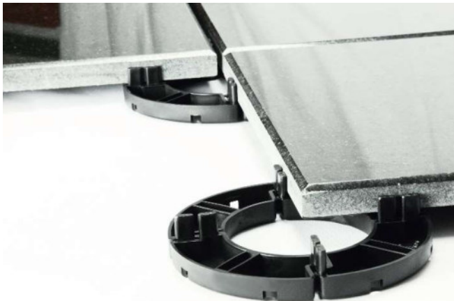
Abb. 23: Starres Stelzlager PP155/15, hier Plattenverlegung mit Kreuzfuge.
