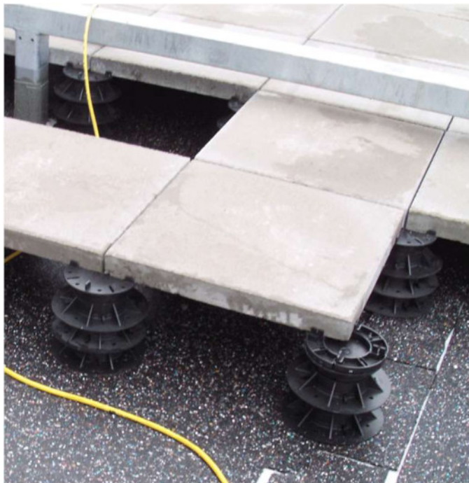
Abb. 17: Höhenverstellbares PLV50/75 mit starren Stelzlagern PP155/15, Bauvorhaben „euro-gate“ Hamburg.
